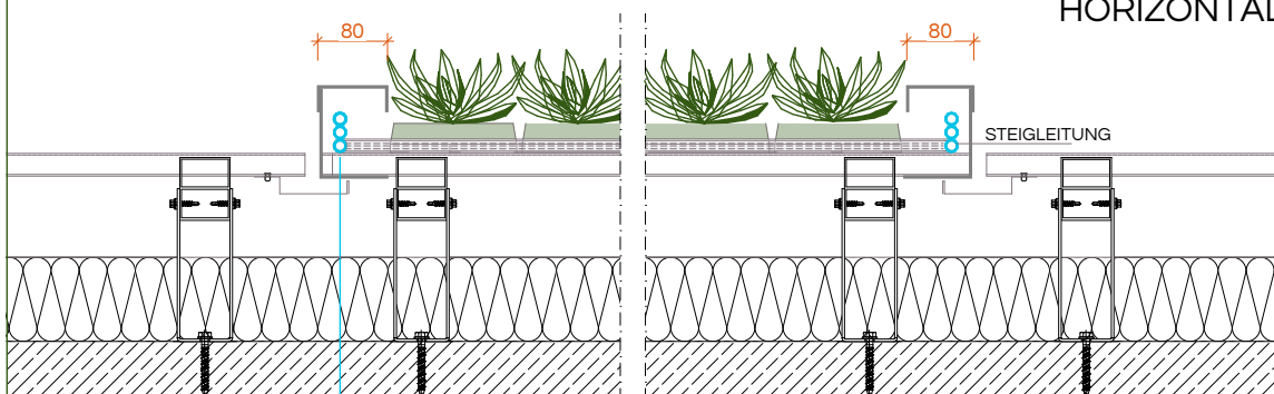
HORIZONTALSCHNITT 1:5
