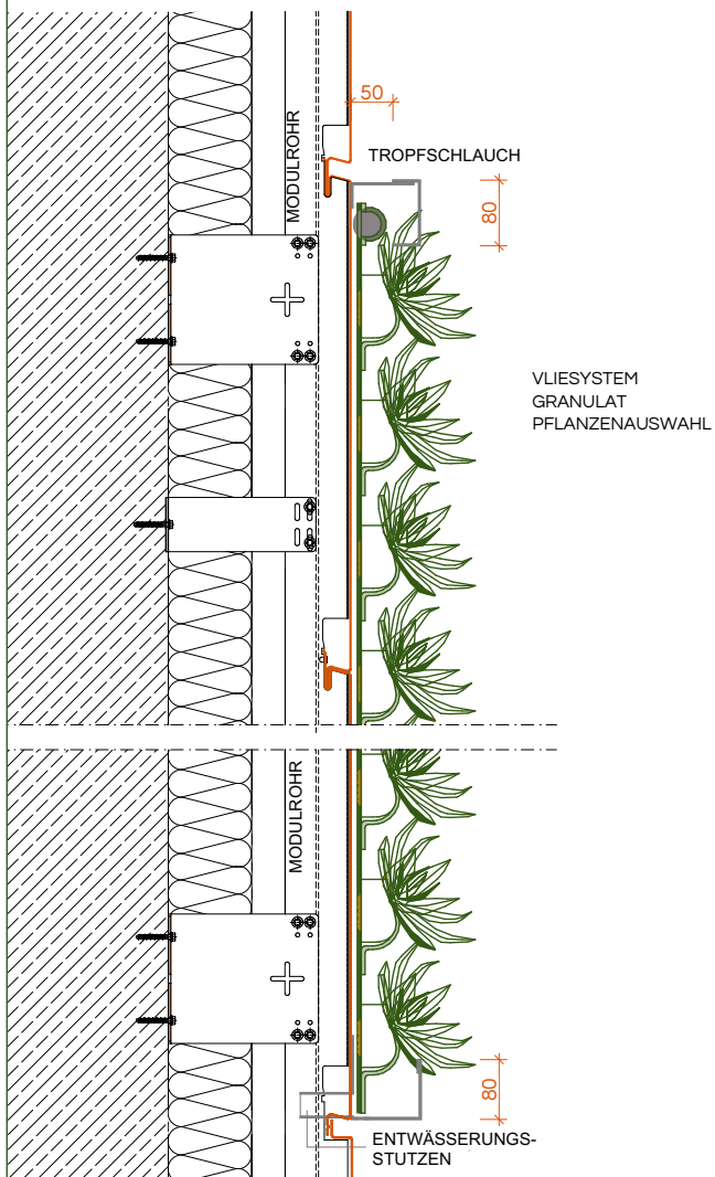
VERTIKALSCHNITT 1:5
